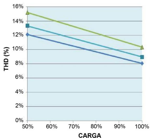
Curva de distorsión armónica
