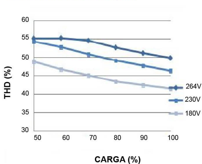
Distorsión Armónica Total (THD)
