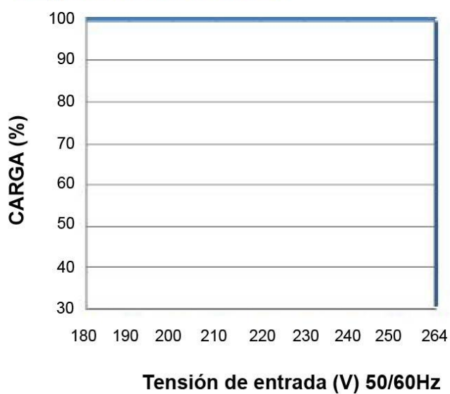
Carga vs Tensión de entrada
