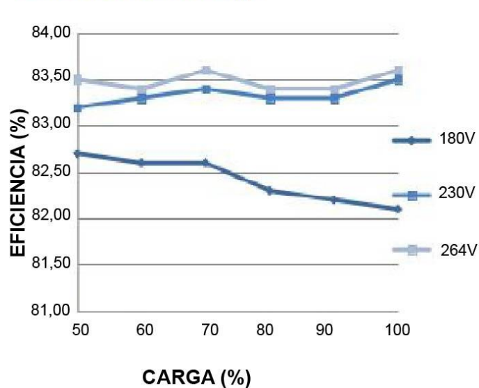
Curva Eficiencia vs Carga
