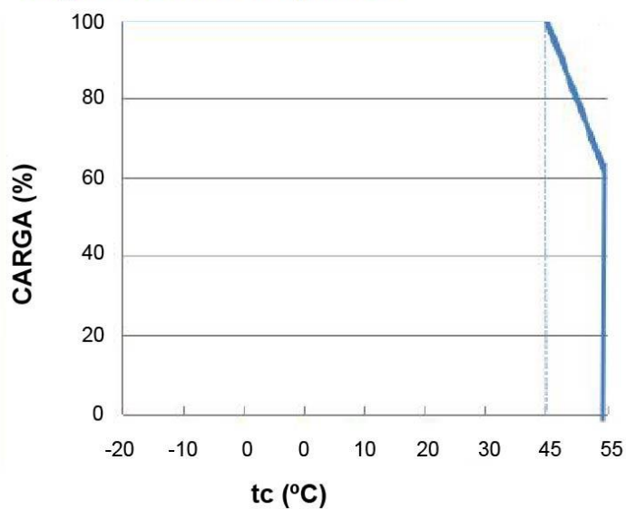
Carga vs Curva de temperatura
