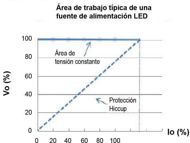
Figura I-V (Área de trabajo)
