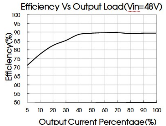
DWLD20-A4815
