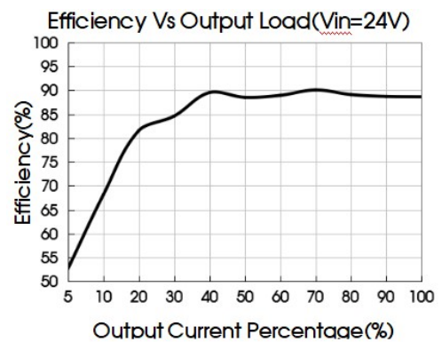
DWLD20-B2405
