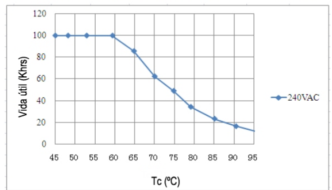
Curva de vida útil vs. temperatura de caja
