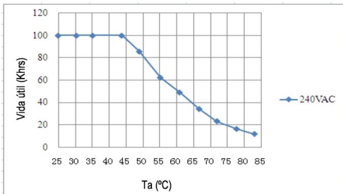
Curva de vida útil vs. temperatura ambiente
