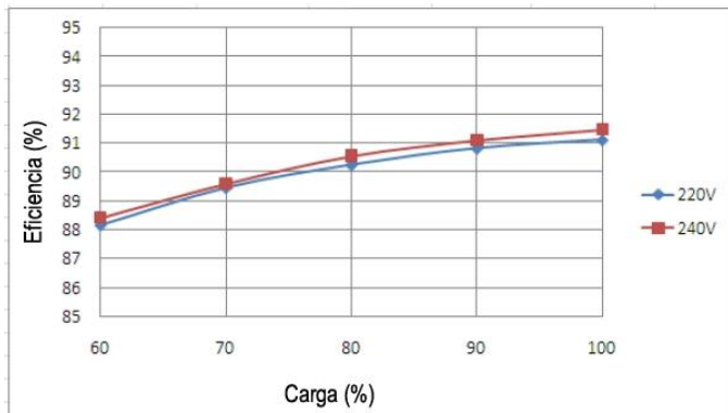
Eficiencia vs. carga para 1400mA
