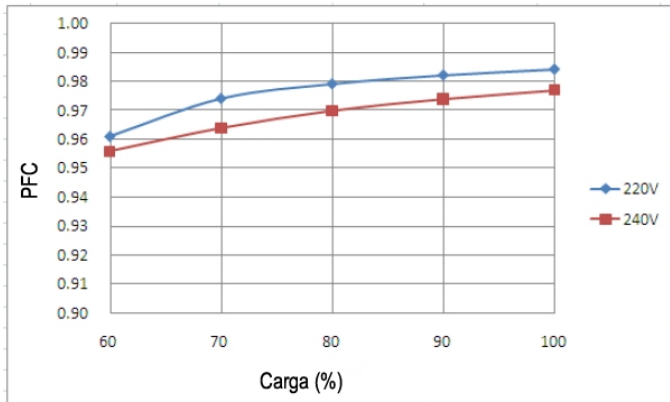
Características PFC para 1400mA
