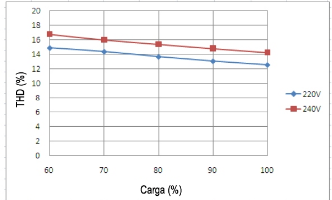
Distorsión armónica vs. carga para 1400mA
