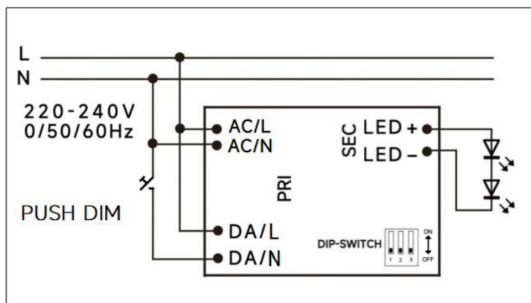
Aplicación Pulsador
