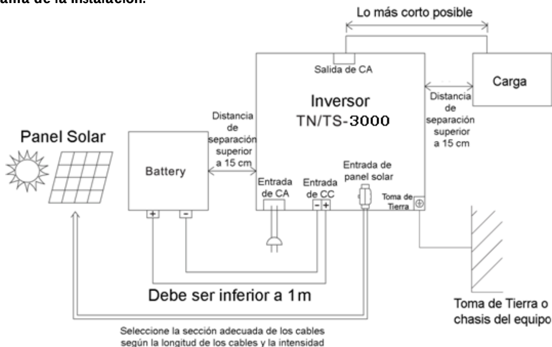
Figura 11 - Diagrama de la Instalación
