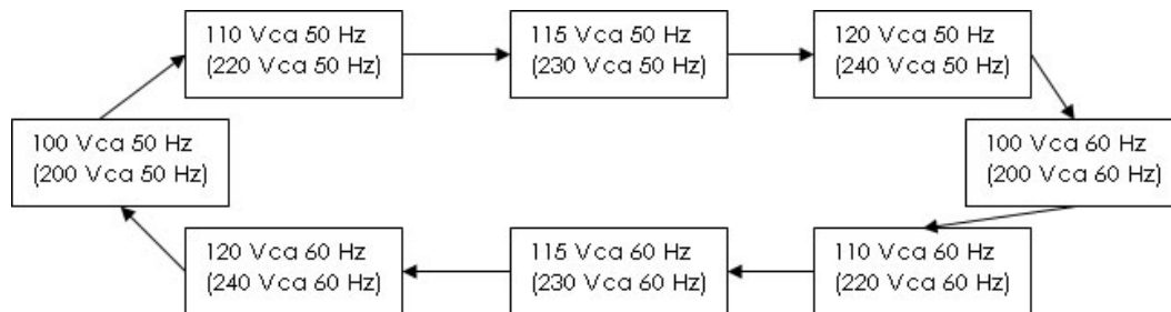
Figura 8 - Diagrama de tensión y frecuencia de salida
