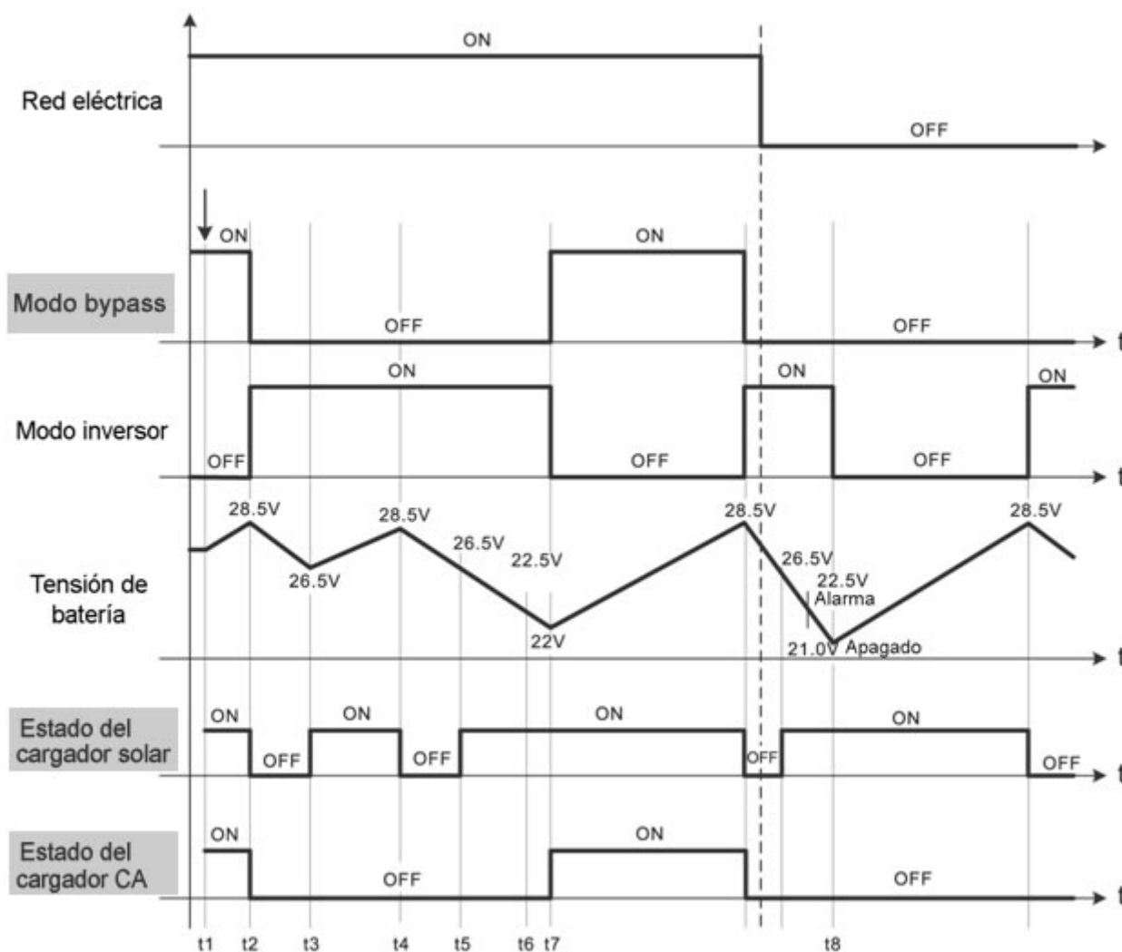
Figura 6 - Explicación del modo de funcionamiento Ahorro de Energía
