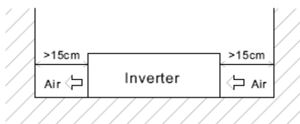
Figura 10 - Ejemplo de Instalación
