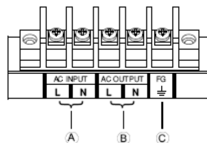
Figura 3 – Terminales de conexión
