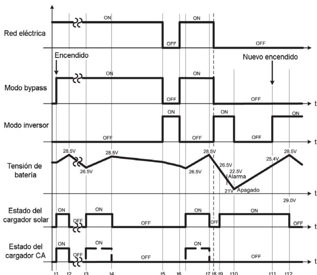
Figura 5 - Explicación del Modo Funcionamiento SAI
