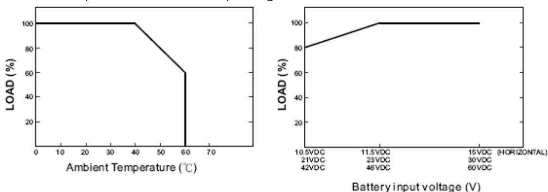
Figura 12 - Curvas de Deriva
