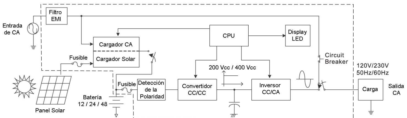
Figura 1 - Diagrama de bloques de Sistema
