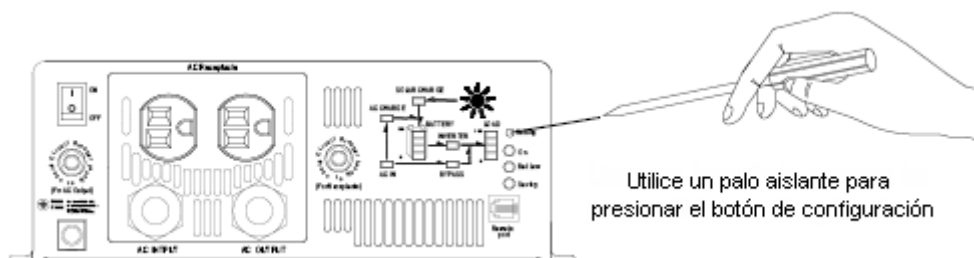
Figura 7 – Ajuste del modo de salida, tensión de salida, frecuencia y modo ahorro de energía
