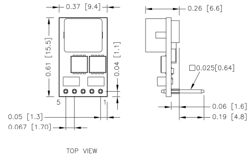
OSR03-12S3P3A
