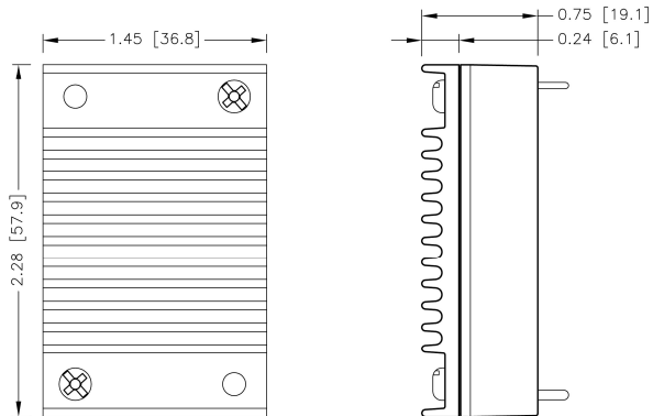
QAE100-□□S□□ -HS 7G-0029B-F
