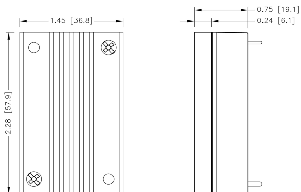
QAE150-□□S□□W -HS2 7G-0031B-F
