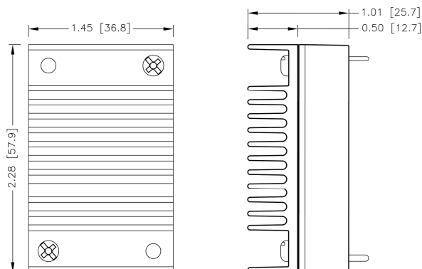
QAE150-□□S□□W -HS1 7G-0030B-F
