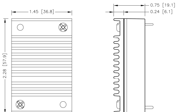
QAE150-□□S□□W -HS 7G-0029B-F
