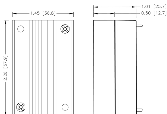
QAE60-□□S□□U - HS3 7G-0032B-F
