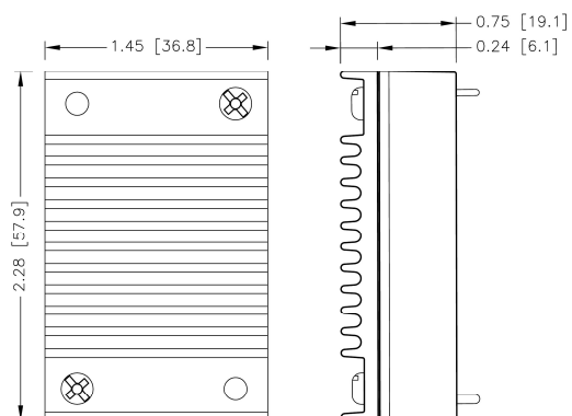
QAE60-□□S□□U - HS 7G-0029B-F
